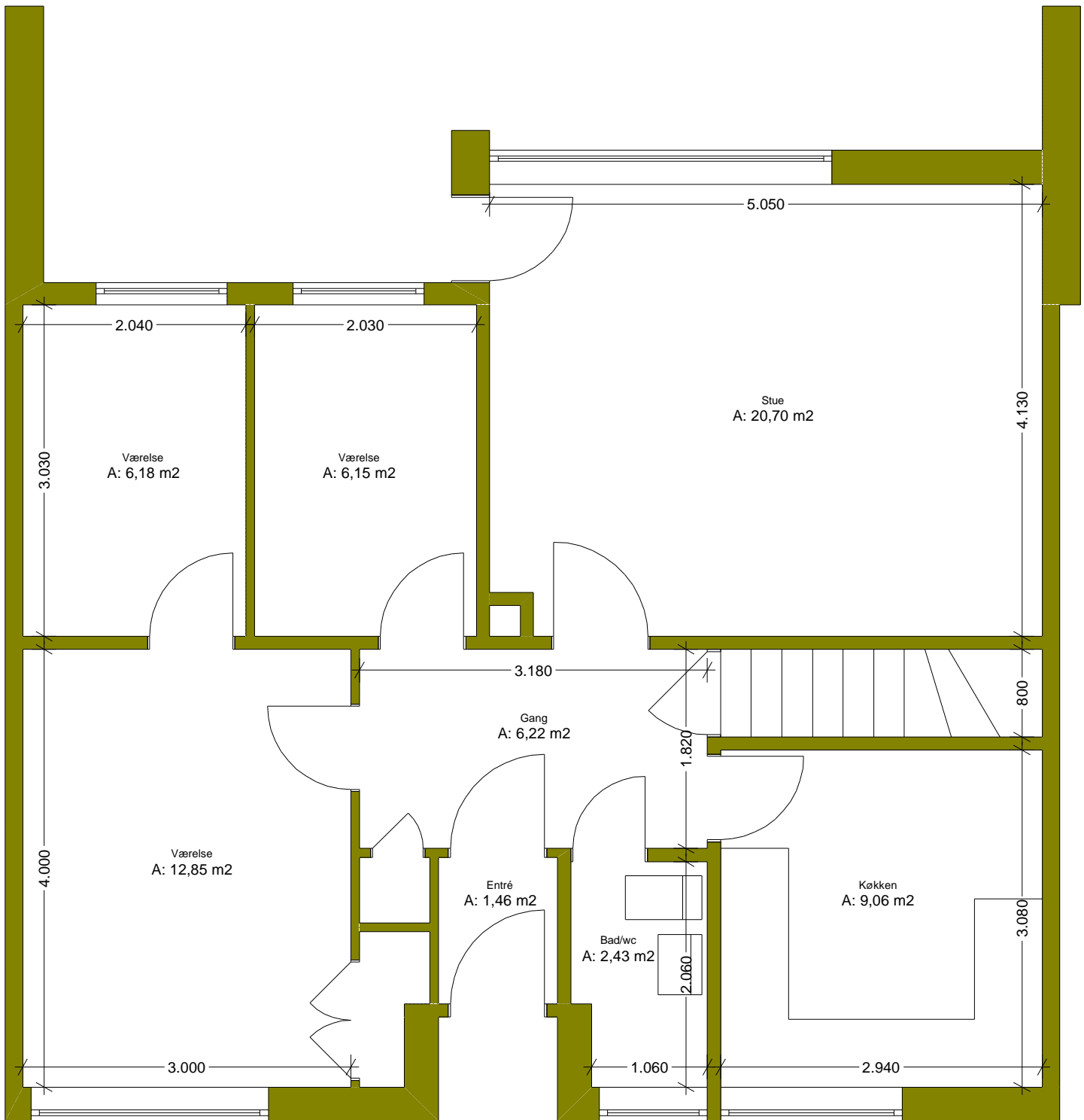
Stueplan
